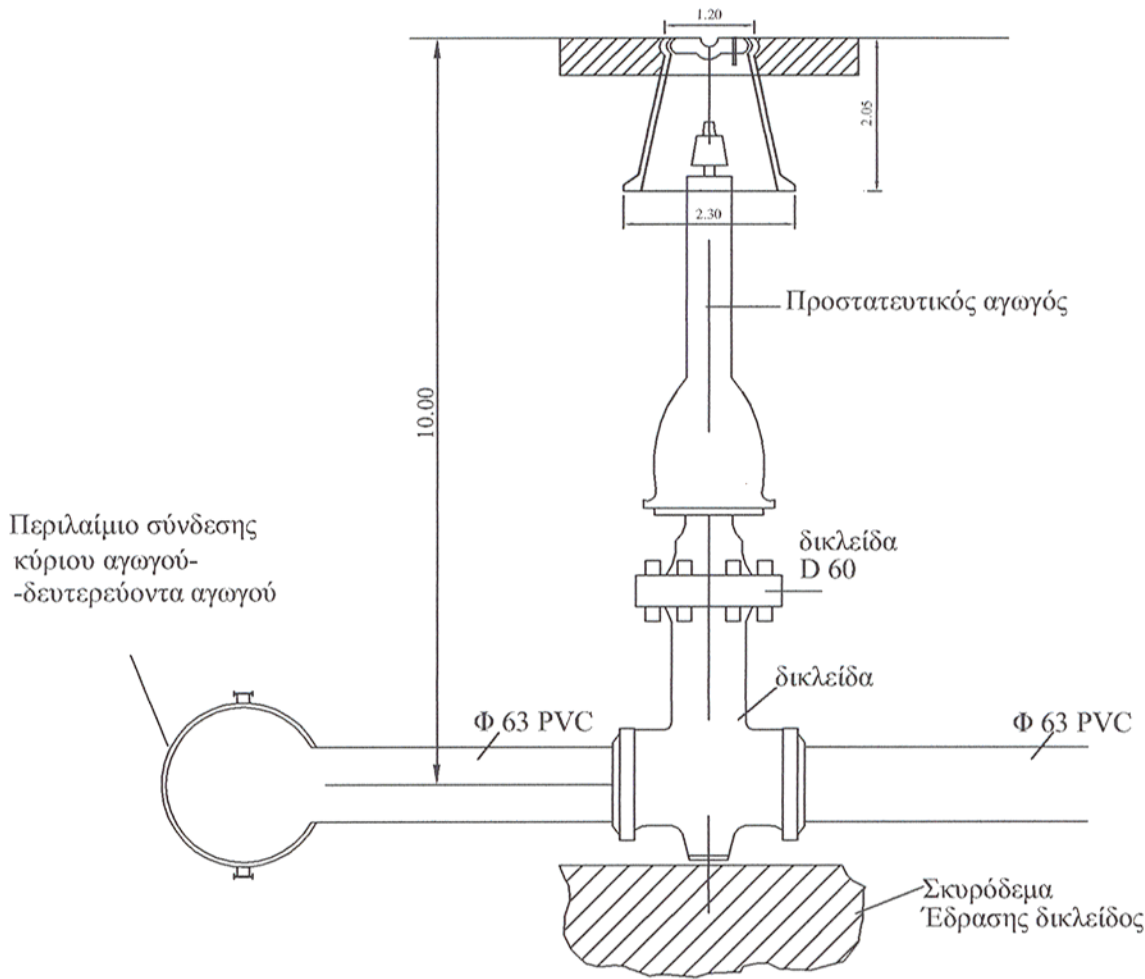
ΚΛΙΜΑΚΑ 1:100 ΛΕΠΤΟΜΕΡΕΙΑ ΚΑΤΑΣΚΕΥΗΣ ΕΜΜΕΣΟΥ ΧΕΙΡΙΣΜΟΥ ΔΙΚΛΕΙΔΩΝ
